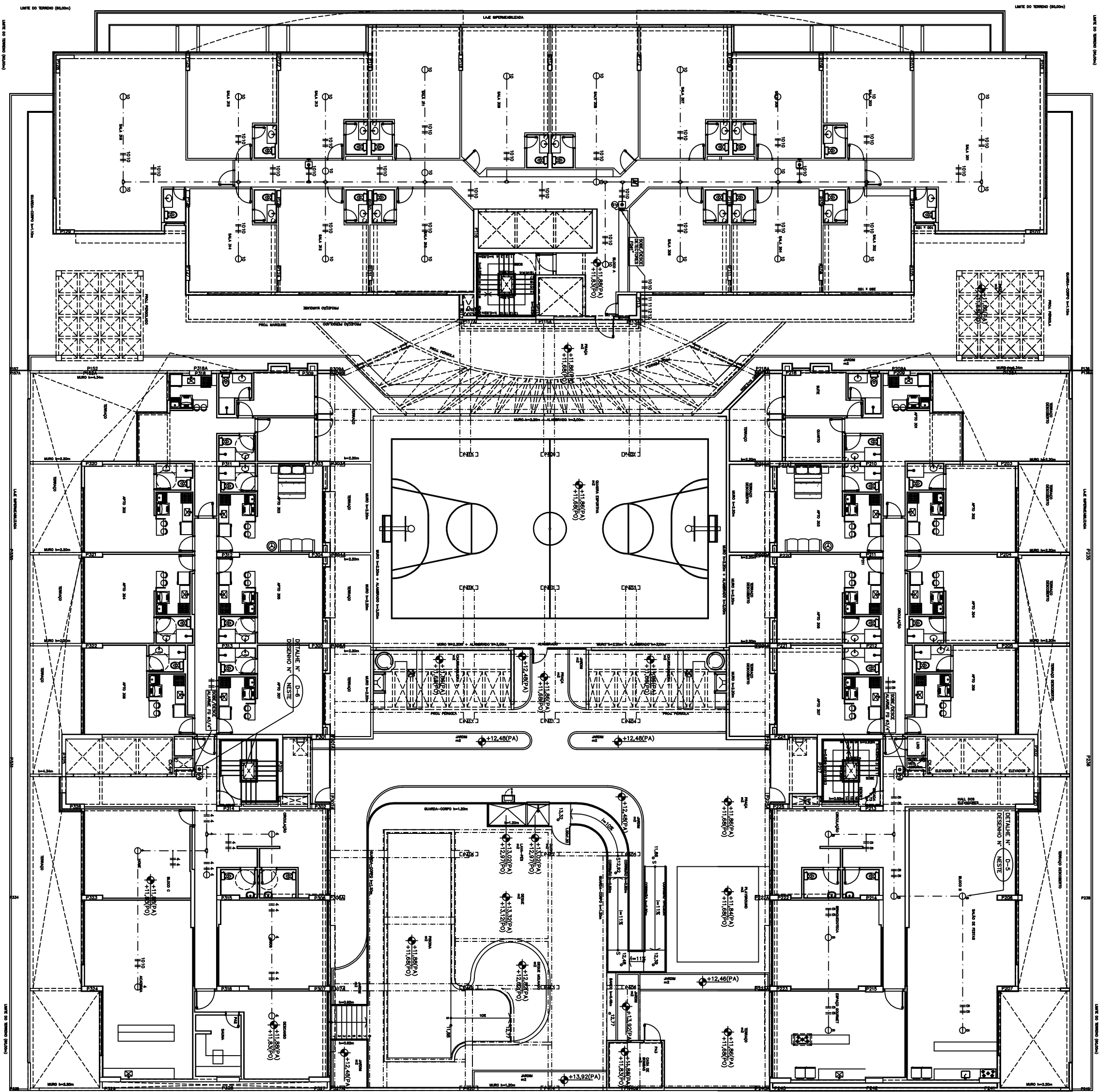
PLANTA BAIXA 3º PAVIMENTO ESCALA 1:100
