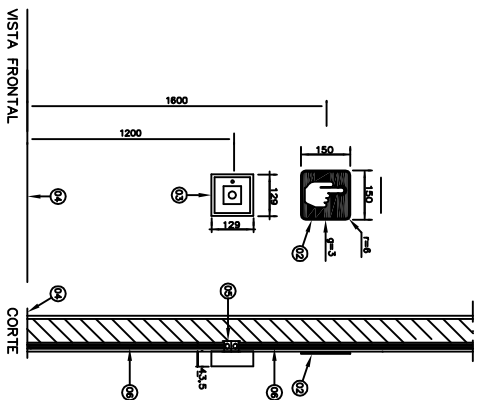
DETALHE D-5 ACIONADOR MANUAL NOS ANDARES TIPO SEM ESCALA
